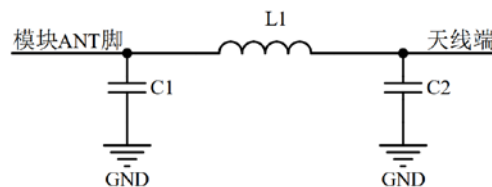
5-2 \pi 型匹配电路
